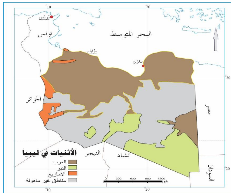
شكل (2) الأثنيات في ليبيا
